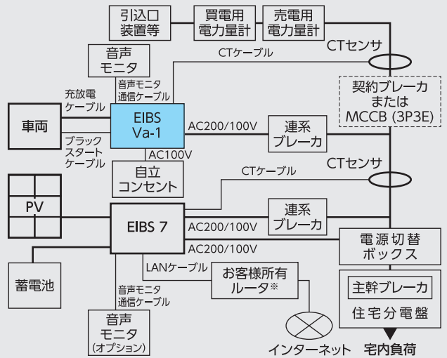
EIBS7 組み合わせ時の接続図
