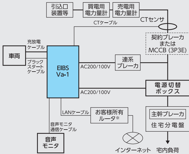
Va-1 単品の接続図
