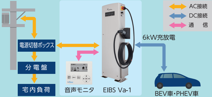
Va-1 単品の接続図
